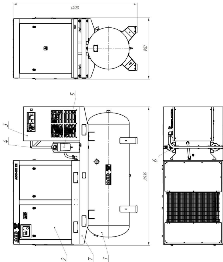
Рисунок 1. Установка компрессорная АСО-БК22М2-ОБ-500 1 – ресивер, 2 – агрегат компрессорный, 3 – осушитель воздуха; 4 – система трубопроводов, 5 – фильтр магистральный АС1041; 6 – фильтр магистральный АС1043, 7 – плита установочная.
