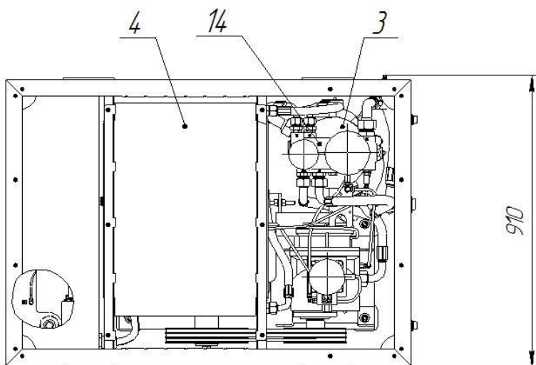
Рисунок 2. Агрегат компрессорный.
