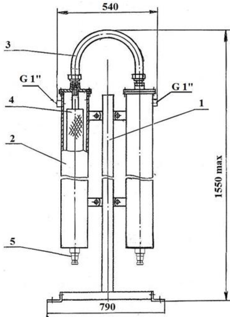
Рис. 2 Фильтрационный модуль ФМ-180/16; ФМ-300/16
