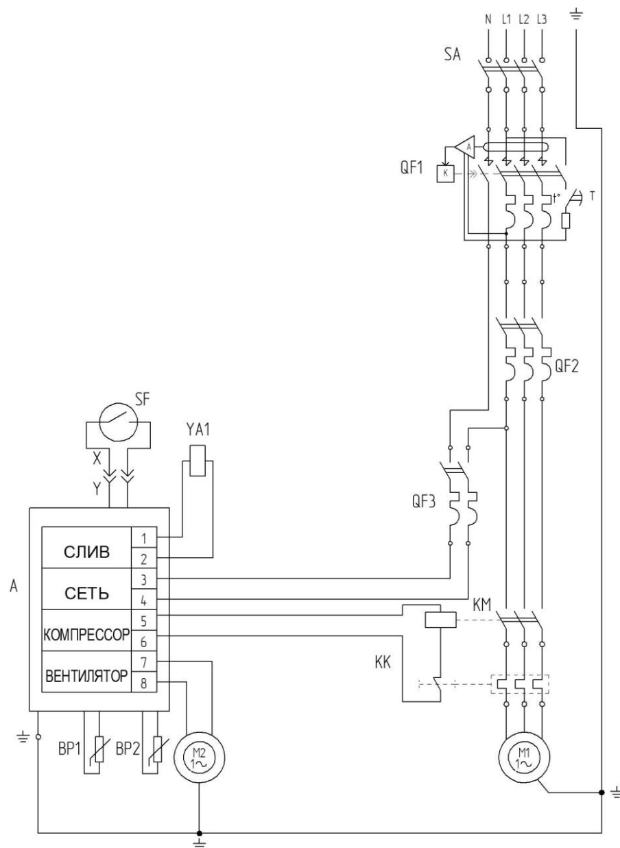
Рисунок 7 – Схема электрическая принципиальная для ОВ-1260.
