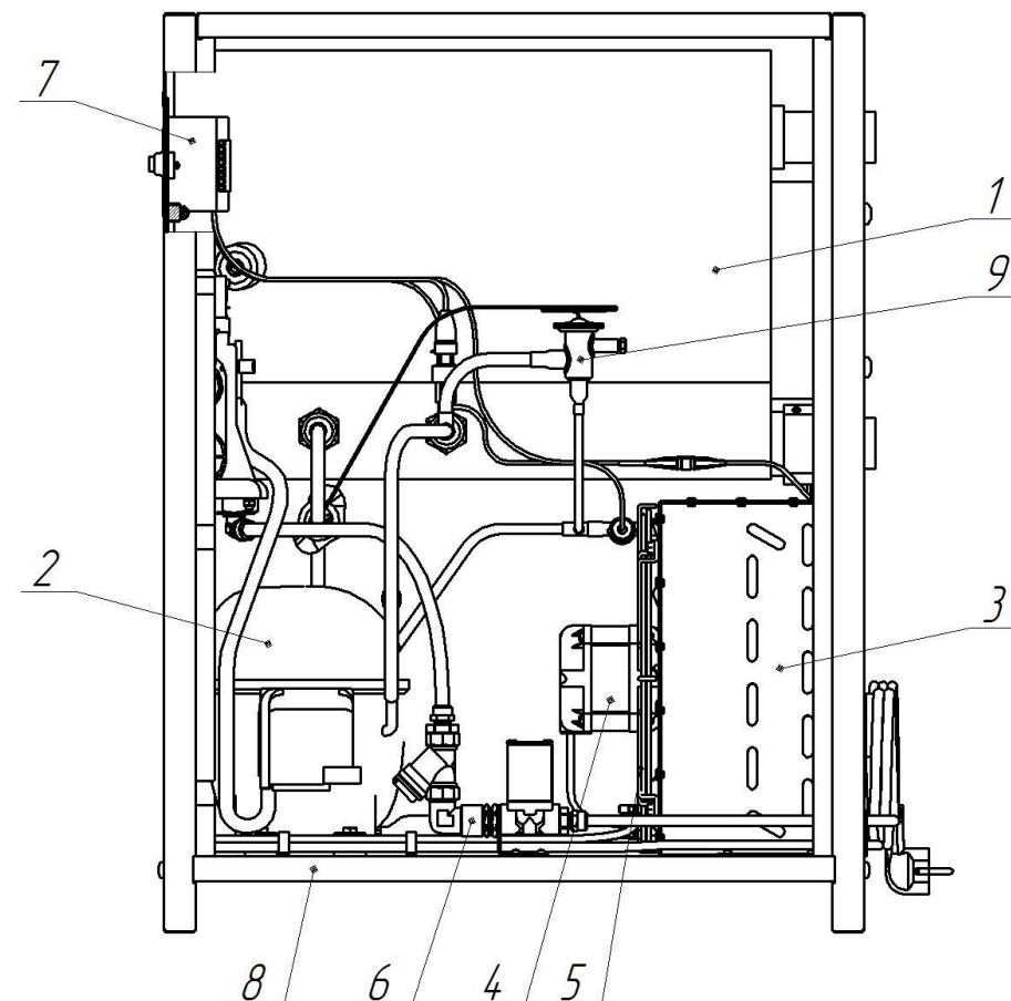
Рисунок 2 – Осушитель сжатого воздуха
