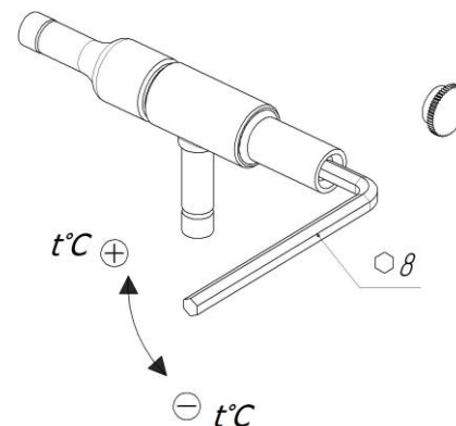
Рисунок 4 – Регулировка регулятора производительности
